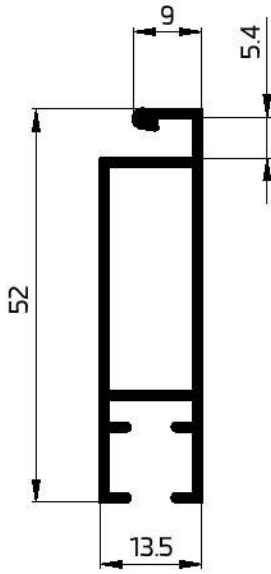
22091 FLY SCREEN 441GR/M T-115mm
