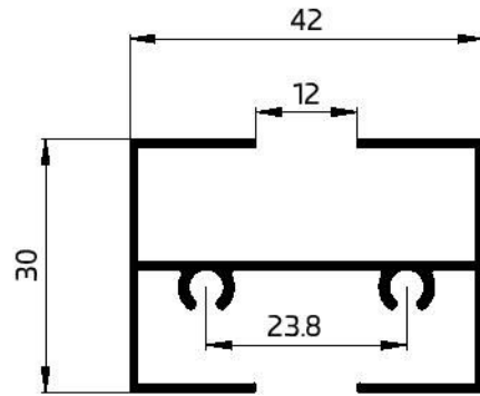
31029 DIVISOR 489.87 GR/M W.T-1mm
