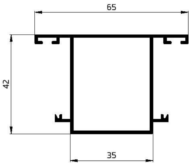
31018 T-SECTION 753.94 GR/M W.T-1.3mm
