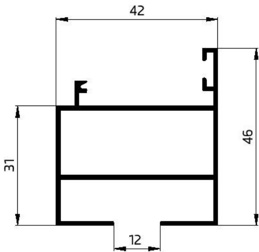
31010 SHUTTER 604.18 GR/M W.T-1.1mm
