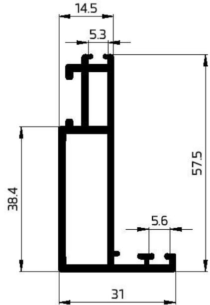
55057 CW-FRAME 767.83 GR/M WT-14 mm
