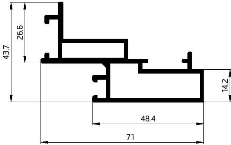
55056 CW-SASH 1041.30 GR/M WT-15 mm
