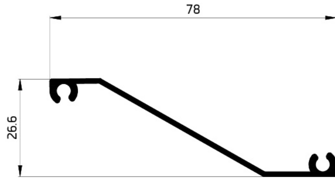
71008 LOUVER 374.20 GR/M W.T-12mm
