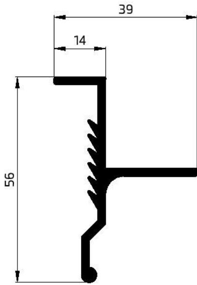
10029 SIGNAGE FRAME 634.12 GR/M W.T - 2 mm
