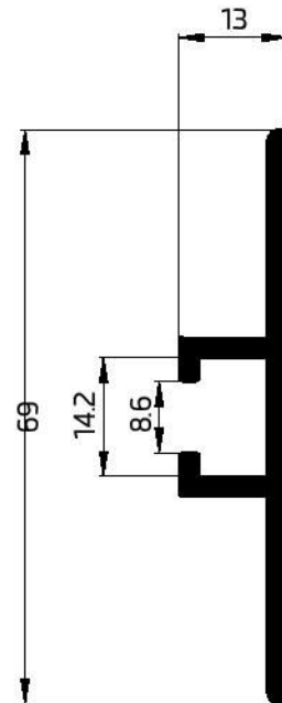
10075 BACK CHANNEL 619.77 GR/M W.T - 2.4 mm
